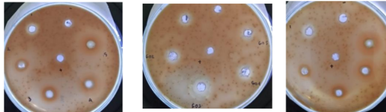
Gambar 3. Zona hambat nanoemulsi minyak lengkuas terhadap H. pylori
