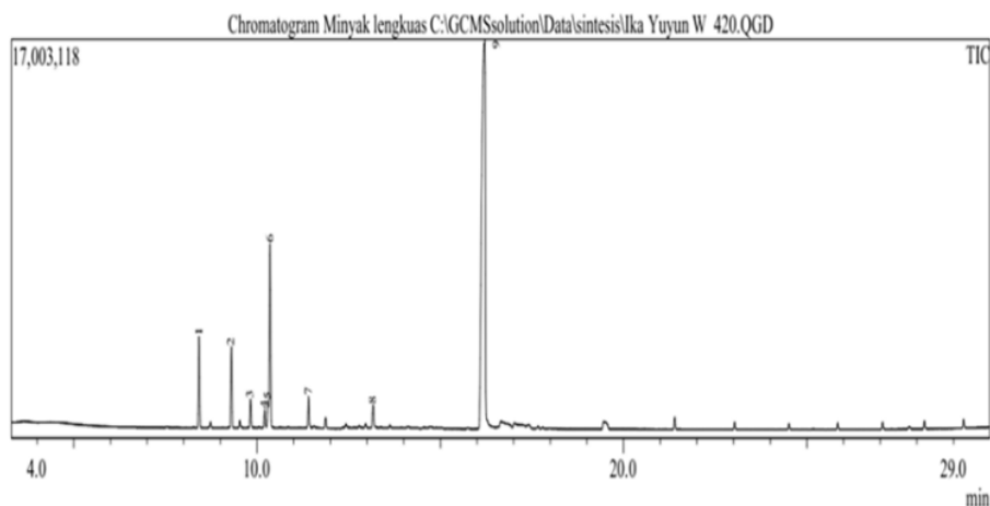
Gambar 1. Hasil kromatogram minyak lengkuas dengan GC-MS
