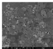
Gambar 1. Produk ZnO-Ag hasil sintesis dengan microwave pada daya 450 W (perbesaran 5000x)
