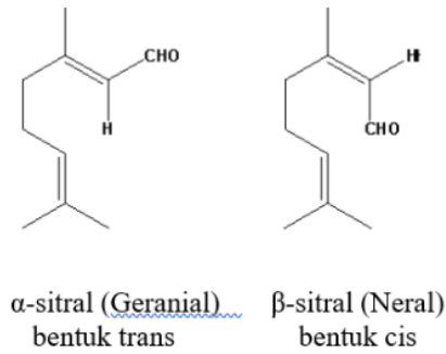
Gambar 4. Struktur senyawa sitral dalam minyak serai dapur
