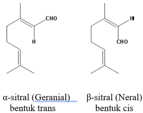
Gambar 4. Struktur senyawa sitral dalam minyak serai dapur
