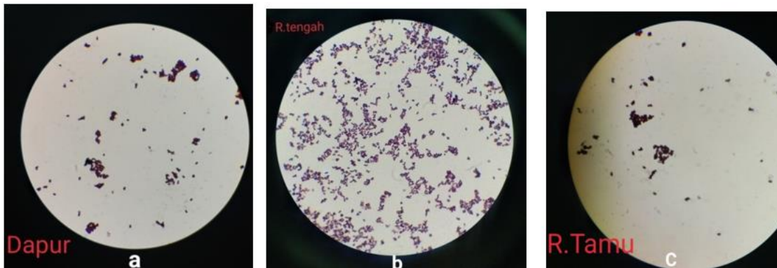
Gambar 1. Pengamatan makroskopis koloni bakteri S. aureus
