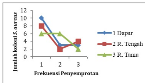
Gambar 4. Hasil rata-rata jumlah koloni penyemprotan minyak peppermint
