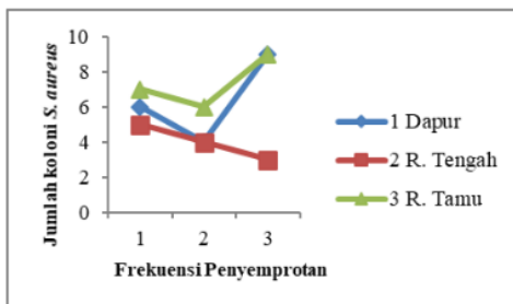
Gambar 5. Hasil rata-rata jumlah koloni penyemprotan desinfektan
