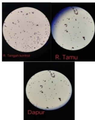
Gambar 1. Hasil uji mikroskopis isolat koloni bakteri
