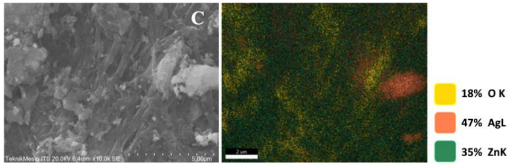
Gambar 7. Hasil analisa SEM-EDX pada nanokomposit ZnO-Ag
