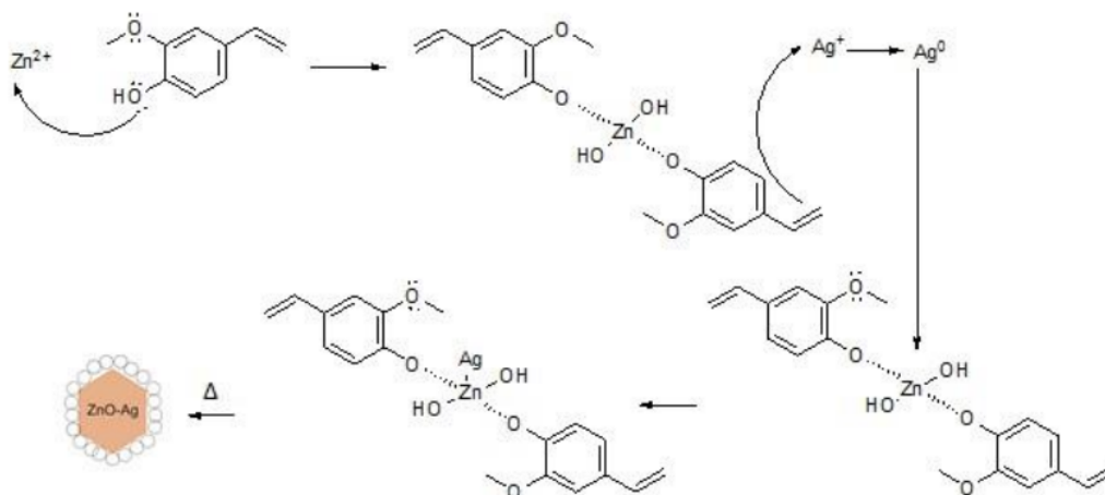
Gambar 6. Mekanisme reaksi nanokomposit ZnO-Ag dengan minyak cengkeh
