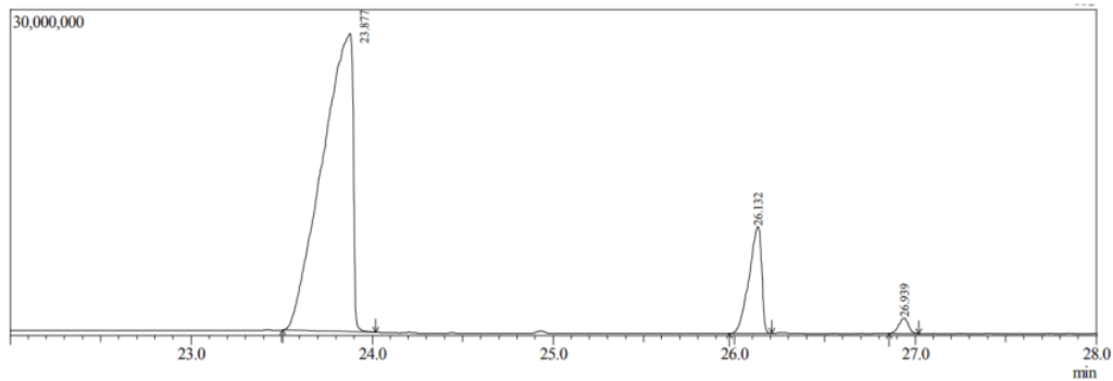
Gambar 2. Kromatogram distilat minyak cengkeh dengan kadar eugenol 73% dengan waktu retensi 23,387
