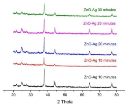
Gambar 4. Hasil analisa difraktogram ZnO-Ag dengan minyak cengkeh
