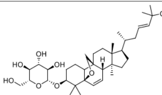
Momordicoside F1
