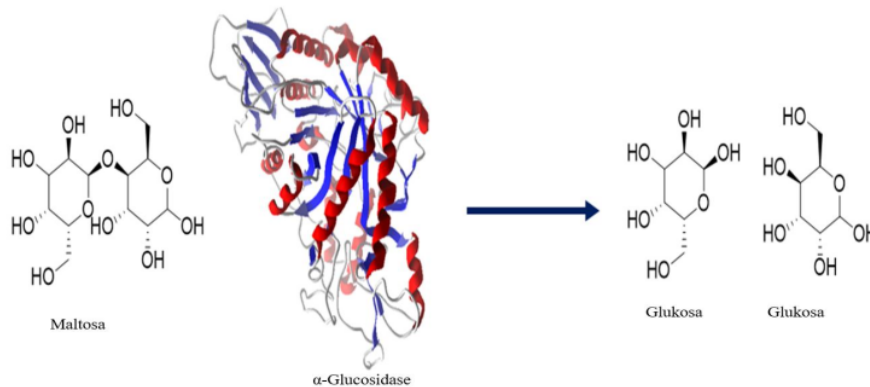
Gambar 3. Mekanisme \alpha -Glucosidase Memecah Disakarida
