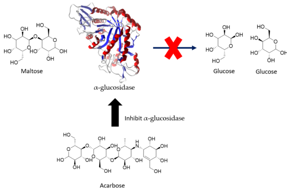
Gambar 4. Mekanisme Acarbose Menurunkan Gula Darah
