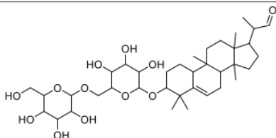
Momordicoside E
