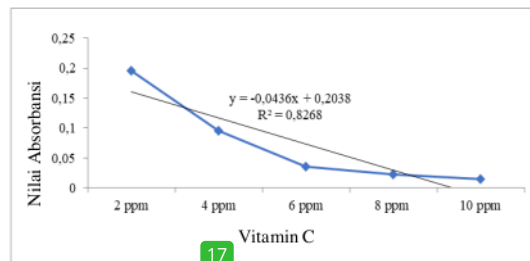
Gambar 1. Kurva Aktivitas Antioksidan Vitamin C Berdasarkan Nilai Absorbansi Menggunakan Metode DPPH
