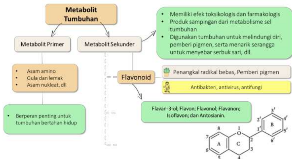
Gambar 14.1. Hasil Metabolisme Pada Tumbuhan Dan Fungsinya Untuk Tumbuhan Dan Makhluk Hidup Lainnya (Manusia); Struktur Kimia Senyawa Flavonoid
