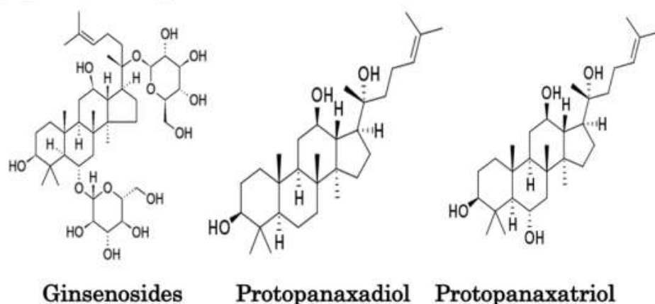
Gambar 16.10 Senyawa Kimia Pada Panax ginseng
