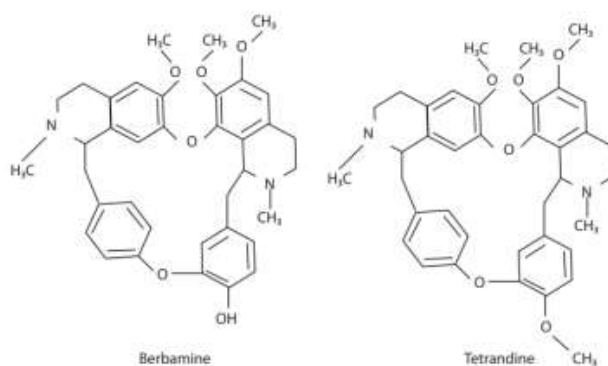
Gambar 12.6. Derivatif alkaloid bisbenzylisoquinoline dengan aktivitas antiinflamasi.
