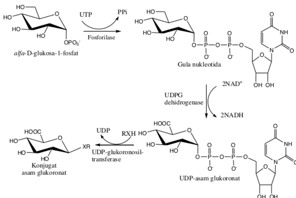
Gambar 16.2 Jalur Biosintesis dan Reaksi UDP-Asam Glukoronat
