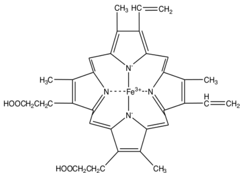
Gambar 16.1 Struktur Heme
